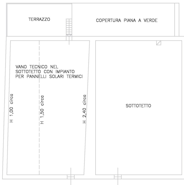
SOTTOTETTO – SCHEMA VISTO DALLA CTU CON ALTEZZE MISURATE GRAAFICAMENTE SUL DISEGNO DEL CONDONO
